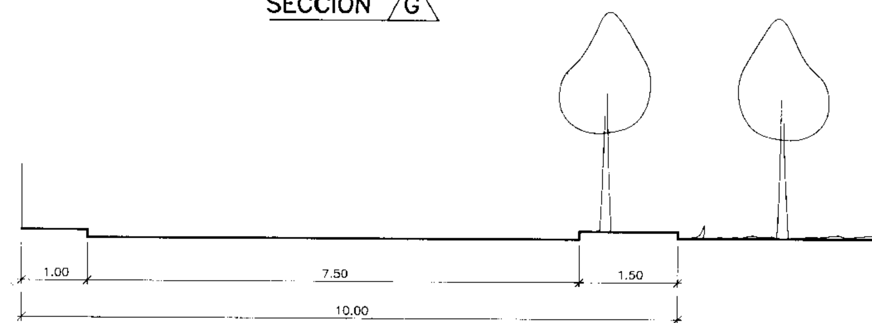
SECCION H
