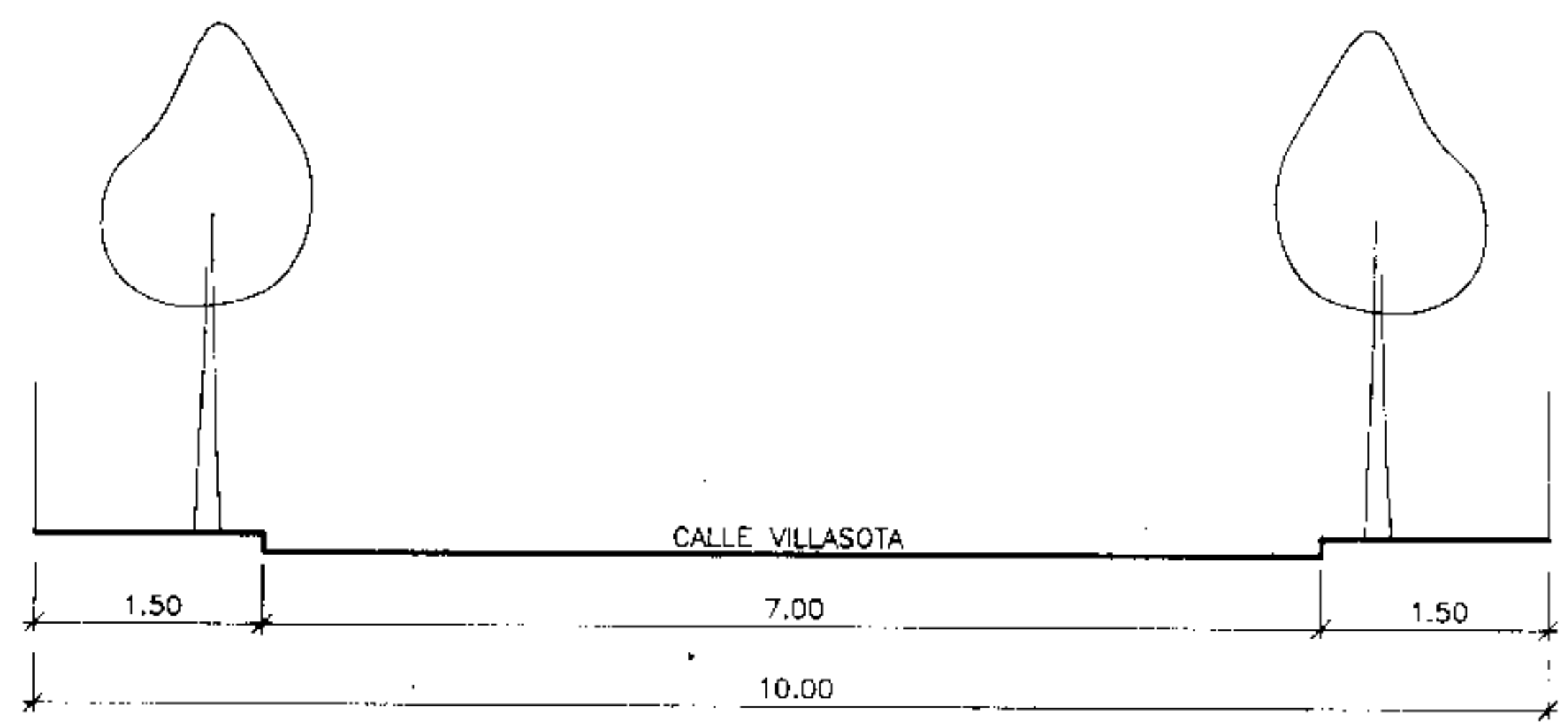
SECCION C
