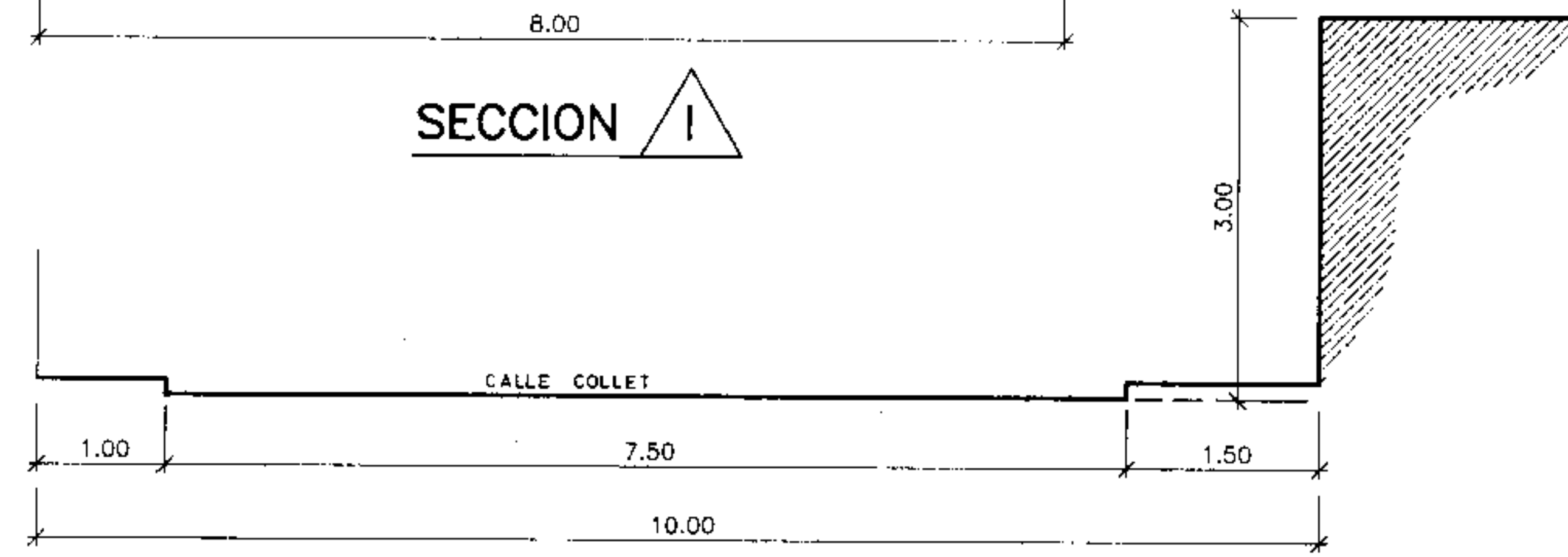
SECCION J
