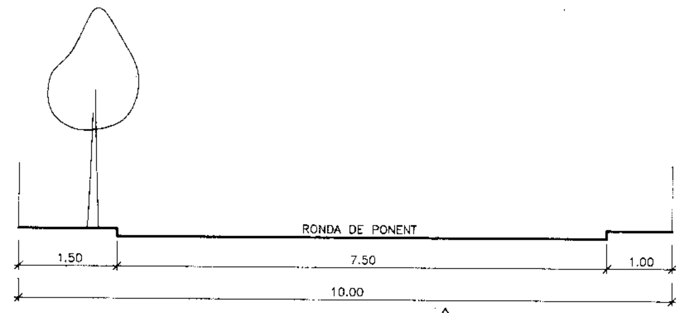
SECCION A
