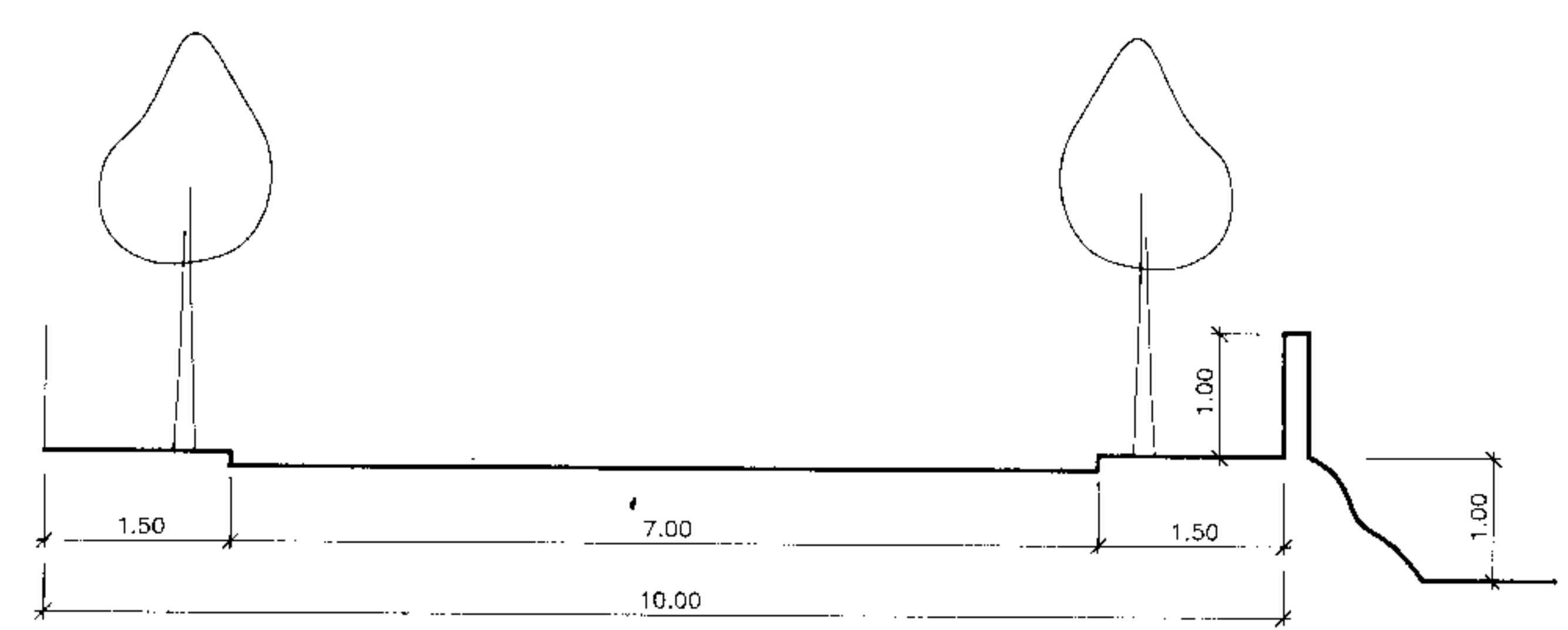
SECCION G
