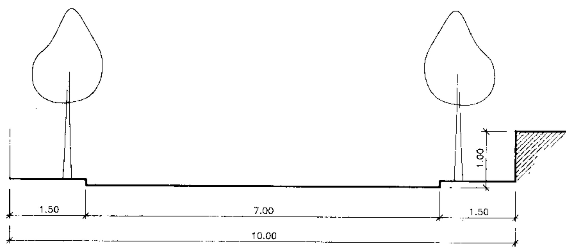
SECCION D
